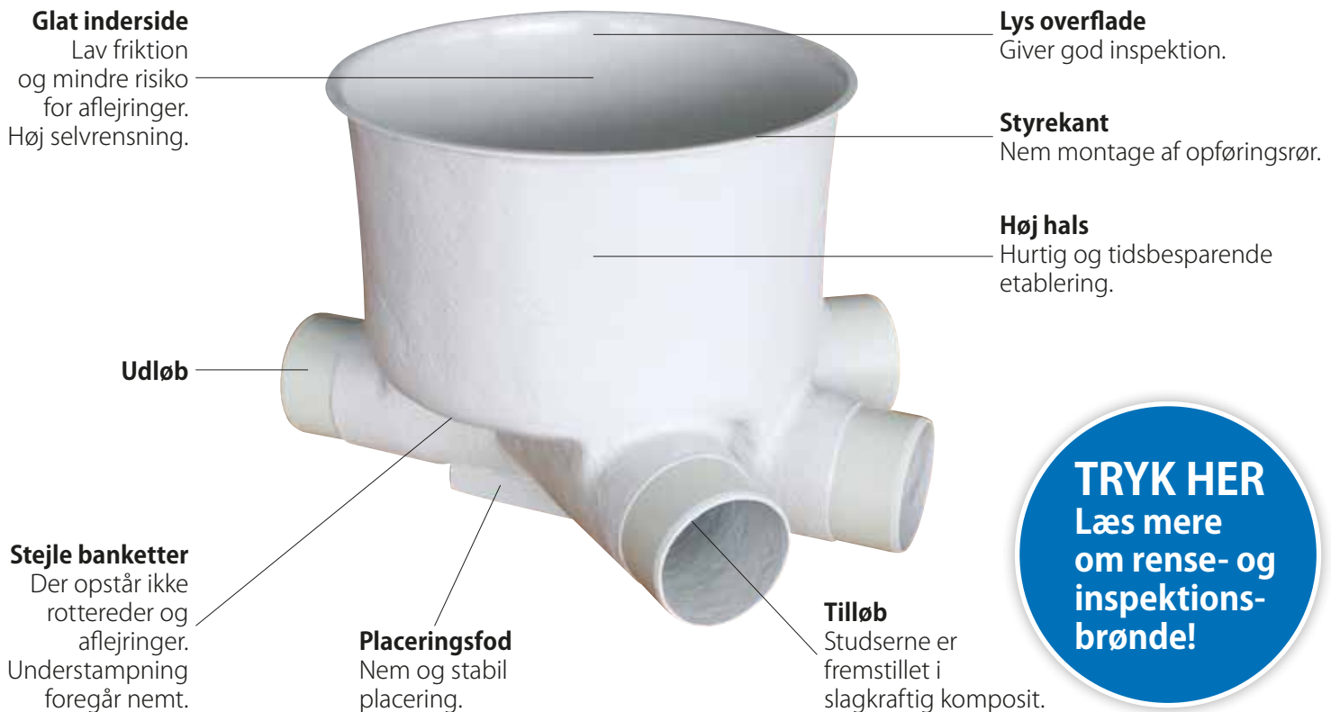
En rens- og inspektionsbrønd giver mulighed for at vedligeholde afløbssystemet uden opgravning
