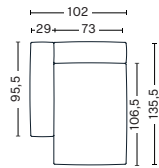
Left armrest Art. S8162 W73/102 x D106,5/135,5 x H37/67 cm Armrest W29 x H67 cm
