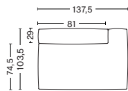
Left backrest Art. S9302 W137,5 x D74,5/103,5 x H37/67 cm
