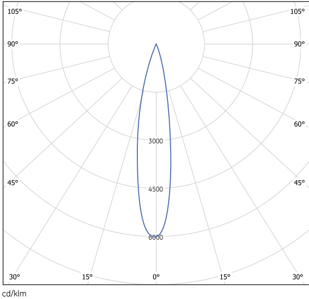
35W CMH-AR111 3000K FL24
