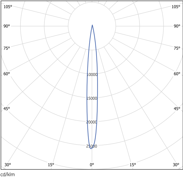
35W CMH-AR111 3000K SP10
