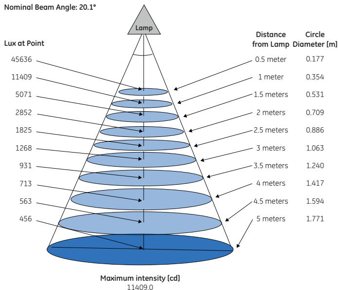
35W CMH-AR111 3000K FL24
