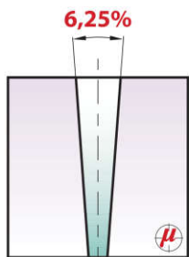
TAPER 6,25% 1:16 CONICIDAD 锥度
