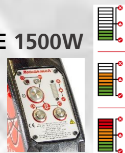
Motorens belastning kan aflæses direkte på displayet
