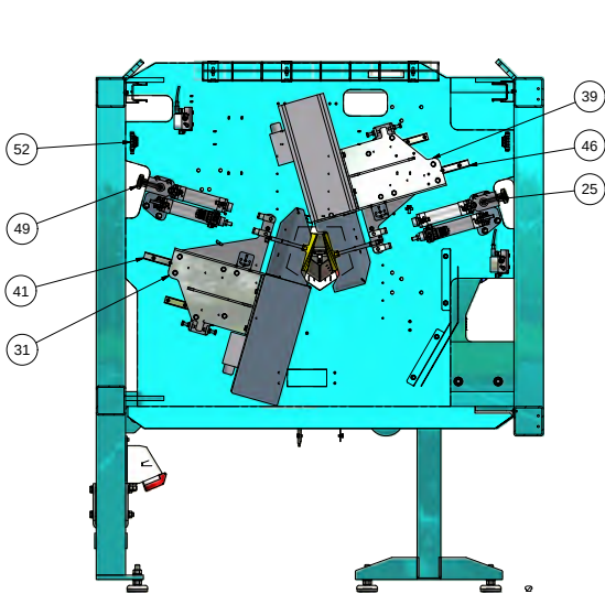
D-D (1 : 10) SET 1
