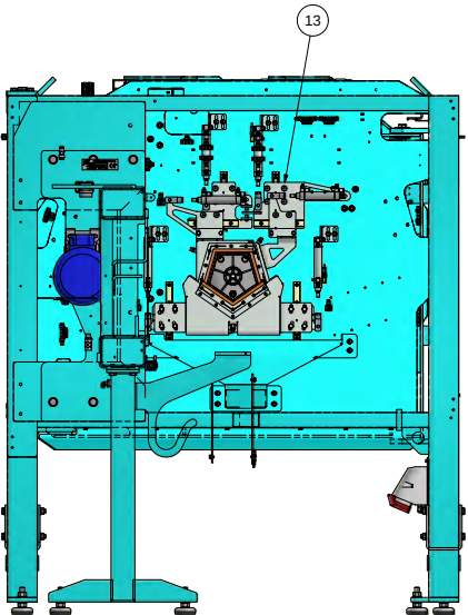
A-A ( 1 : 10 ) Beam washer
