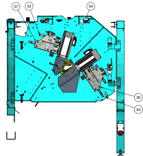
F-F (1 : 10) SET 4
