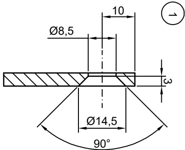
Schnitt A-A
