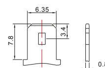
F2 Terminal
