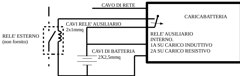
Esempio di schema di collegamento con utilizzo del relè ausiliario interno al caricabatteria. Il relè ausiliario è Normalmente Chiuso e commuta all'accensione del caricabatteria. Il relè ausiliario interno può essere utilizzato con correnti massime di 1A su carico induttivo oppure 2A su carico resistivo.
