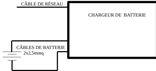
Exemple de schéma de connexion entre chargeur de batterie et batterie.
