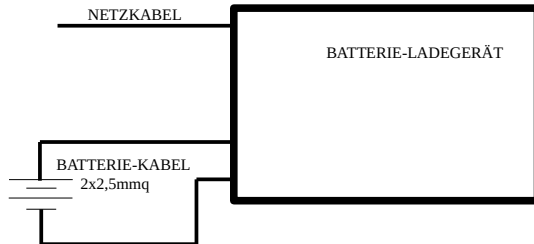
Beispiel für Anschluss-Schaltplan zwischen Batterie-Ladegerät und Batterie.
