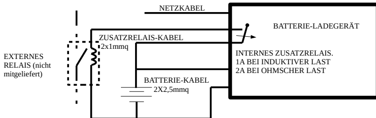
Beispiel für Anschluss-Schaltplan mit Verwendung eines Zusatzrelais im Batterie-Ladegerät. Das Zusatzrelais ist normalerweise geschlossen und schaltet sich beim Einschalten des Batterie-Ladegeräts um. Das interne Zusatzrelais kann mit Höchststromwerten von 1A induktive last oder 2A ohmsche last verwendet werden.
