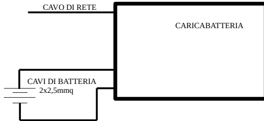
Esempio di schema di collegamento tra caricabatteria e batteria.
