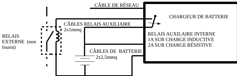
Exemple de schéma de connexion avec l'emploi du relais auxiliaire interne du chargeur de batterie. Le relais auxiliaire est Normalement Fermé et commute l'allumage du chargeur de batterie. Le relais auxiliaire interne peut être utilisé avec des courants maximums de 1A au inductive charge or 2A au résistif charge.
